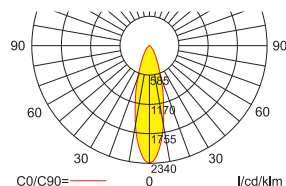
Lampenlichtstrom / Luminous flux: 280lm
