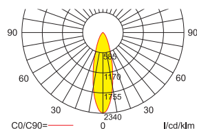
Lampenlichtstrom / Luminous flux: 120lm
