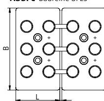
Abb. C Baureihe OPzS
