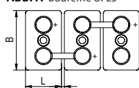
Abb. A Baureihe OPzS
